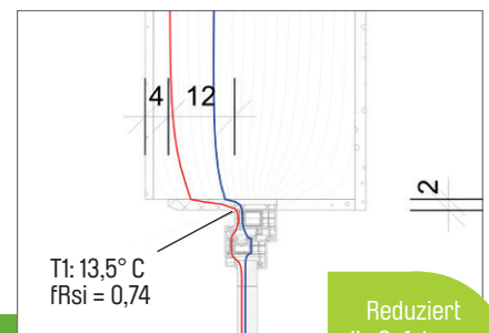
Optimierter Isothermenverlauf mit I-LP therm
